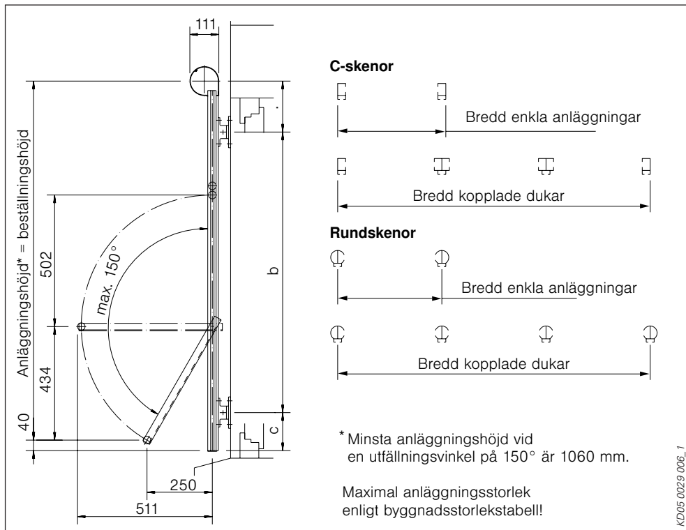
bild 339: Måttanvisning markisolett typ 109
